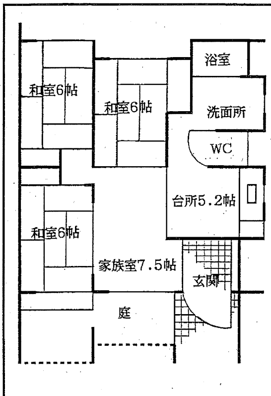
N棟 1 階
