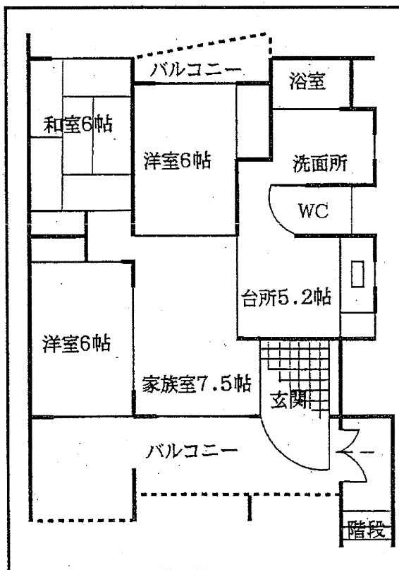
N棟 3 階
