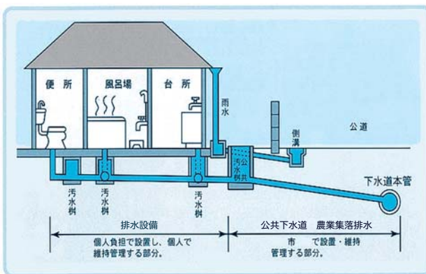
（雨水は既設の側溝や水路に流すことになり、汚水管には流入できません（分流水道））
