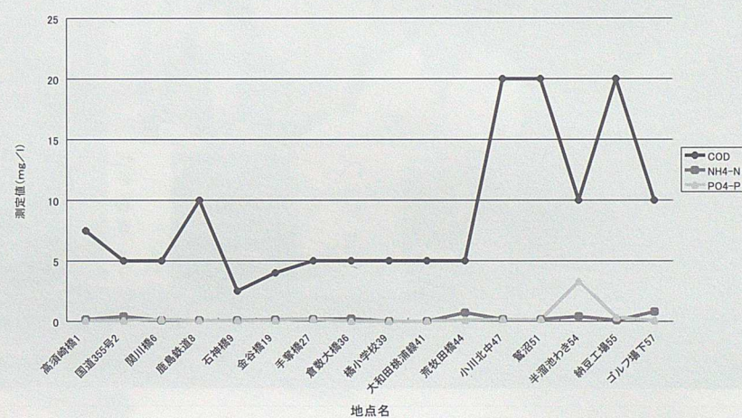
梶無川本流のCOD・NH4-N・PO4-P
