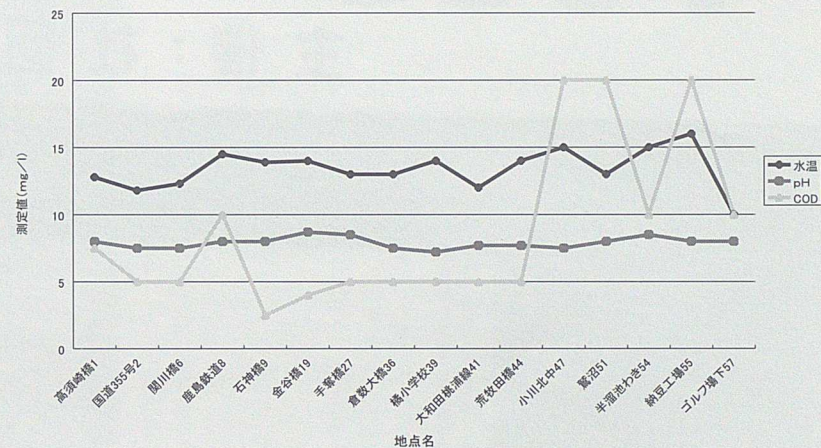
梶無川の本流の水温・pH・COD
