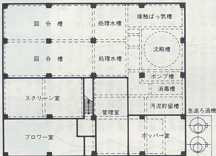
■ 施設平面図(1F)
