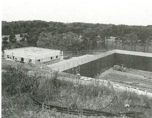
工事が進められている最終処分場
