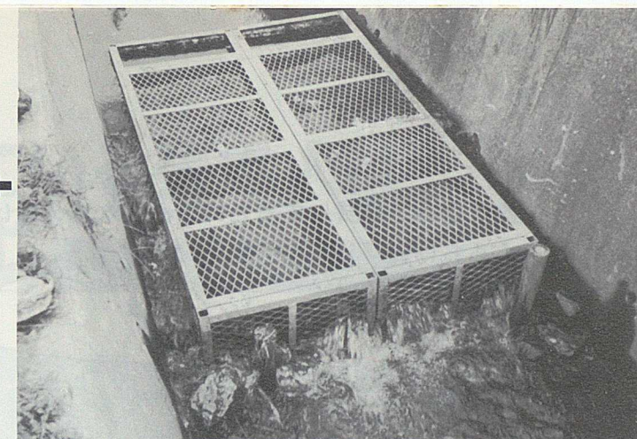
設置した木炭浄化施設
