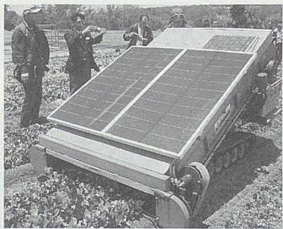
↑収穫機（ソーラーパネル付きでバッテリーをつけ改良して使用している）
