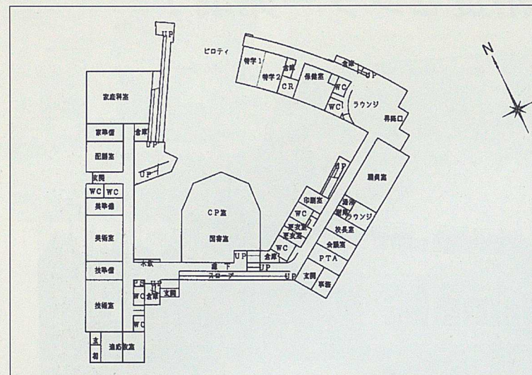
●平面図（2F）
