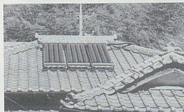
真空管形集熱器（熱媒 水・不凍液） 真空で放熱を防ぎ、高温集熱ができる。
