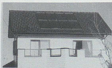
平板形集熱器（熱媒 水・不凍液） 選択吸収膜を用い集熱効率を高めた。
