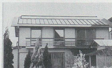
空気式集熱器 ガラスなし集熱面で予熱し、ガラス付集熱面で高い温度にする。
