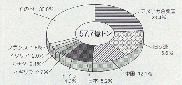
化石燃料の燃焼による国別CO 2 発生量(1992年)
