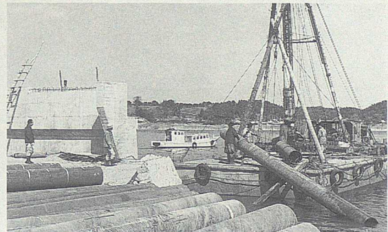
鹿行大橋の橋脚のためのパイルが打ち込まれる
