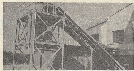
▲焼却炉の灰はハイバンカーに集められ埋立地へ
