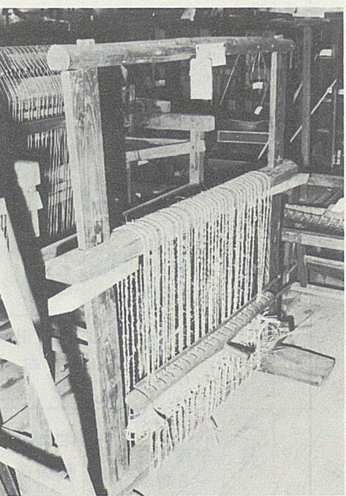
▲ 昭和以前の2人で織るむしろ織機
