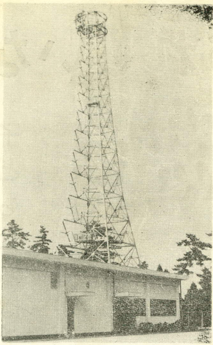
建設すむ北浦受信所。地上40mの連絡鉄塔も完成。この上に間もなくパラボラアンテナが付き、これを通して、本社との連絡や遠隔操作が行なわれる。
